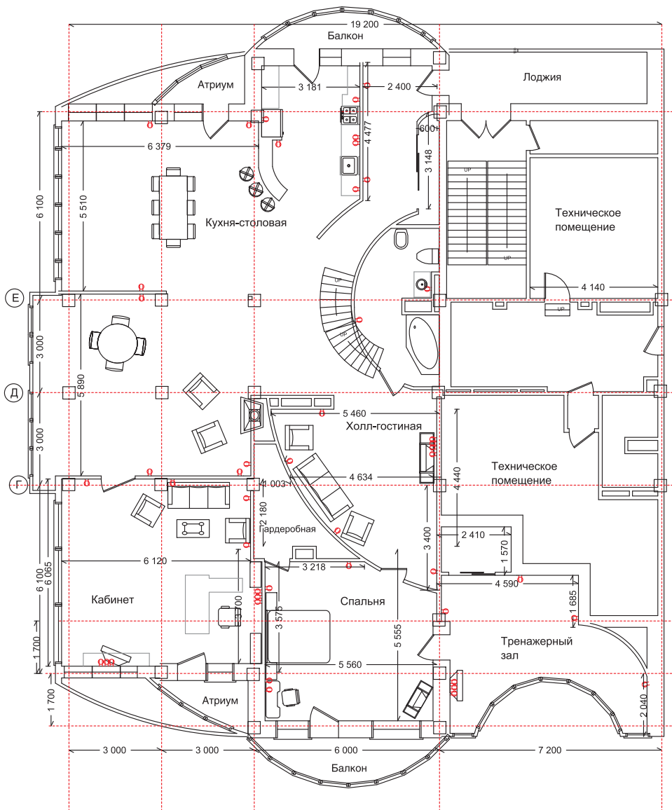
План 14 этажа (1 уровень) пентхауса «Звездочет» в жилом комплексе «Вертикаль» по улице Мира, 282
